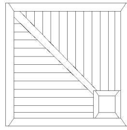
2. Carré - 2 pentes - Siphon en angle
