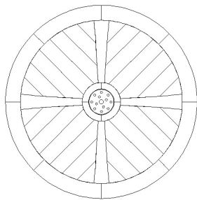
5. Circulaire - 4 rayons - Siphon central
